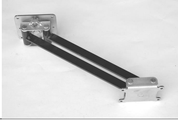
DSK-19 Servis Masası Dönme Mekanizması/ Service Table Swivel Mechanism
