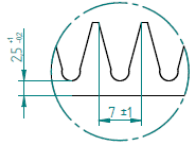
EINZELHEIT B
